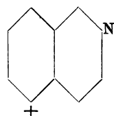
\delta Säure oder Dahlsche Säure.
